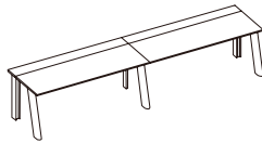
Single Bench w/A-Shape Mid-leg for 2 People 单边共享台带A形中脚: 2人 W: 2400^, 2800, 3000, 3200, 3600 D: 800, 900, 950 H: 725
