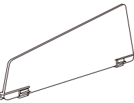
Asymmetric Frameless Screen - Fabric, PET, MFC 不对称无框屏风 - 布料, PET, 三聚氰胺板 W: 1200, 1400, 1500, 1600, 1800 H: 455
