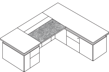
Executive Desk, w/Extended Drawer Cabinet W3800 D2800 H760 W3600 D2800 H760 W3400 D2600 H760 W3200 D2600 H760 W3000 D2400 H760 W2800 D2400 H760 W2400 D2200 H760
