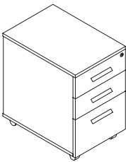
Mobile Pedestal (3 drawers) 三抽活动柜 W: 380 D : 550 H : 600
