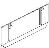
Metal Modesty Panel Fixed on Top 金属前挡板，台底固定 W: 900, 1100, 1200, 1300 T: 12 H: 320
