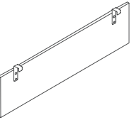
MFC Modesty Panel Fixed on Top 三聚氰胺板前挡板，台底固定 W: 940, 1140, 1240, 1340 T: 16 H: 350
